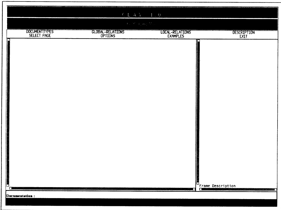
Abbildung 6.16: Der Initialzustand
