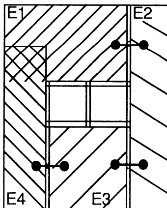
Abbildung 4.11: Globale Konsistenz
